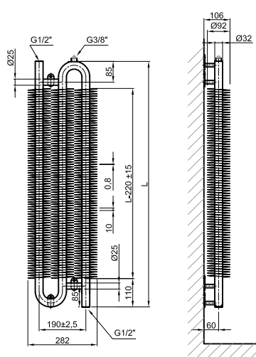
RA03 32×2×92 VERTICAL RIGHT
