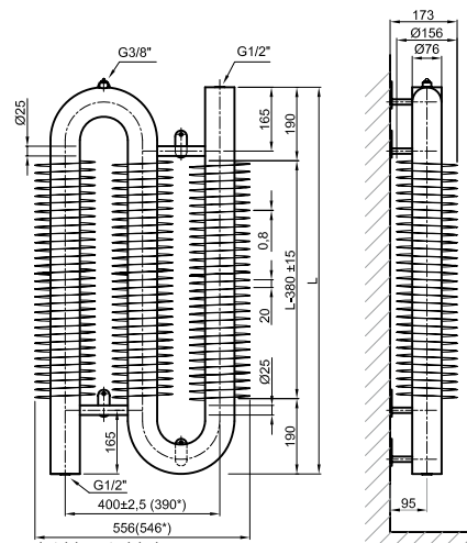
RA03 76×2,5×156 VERTICAL LEFT
