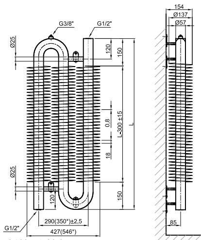
RA03 57×2,5×137 VERTICAL LEFT
