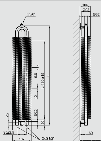
RA02 32×2×92 VERTICAL
