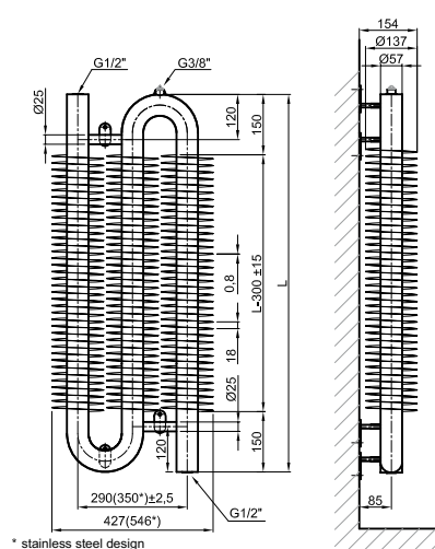
RA03 57×2,5×137 VERTICAL RIGHT
